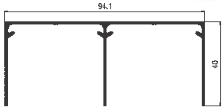
DINTEL MARCO ADR-511 peso: 810 grs/mt.
