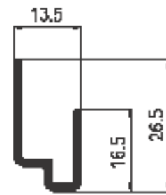
ZOCALO DINTEL HOJA ADR-513 peso: 210 grs/mt.
