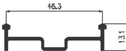
GUÍA de MARCO ADR-512 peso: 321 grs/mt.
