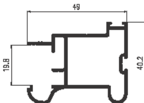
PARANTE de HOJA ADR-1888 peso: 709 grs/mt.
