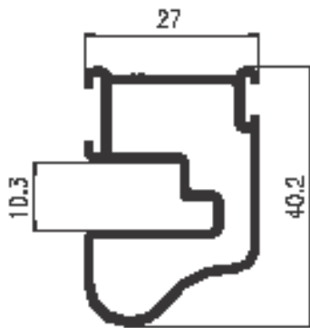
PARANTE de HOJA ADR-510 peso: 548 grs/mt.
