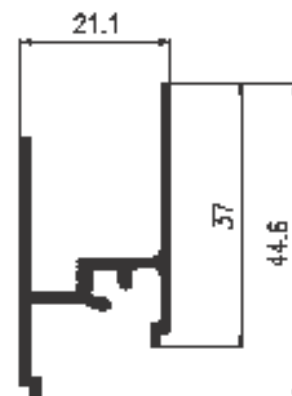
ZOCALO DINTEL HOJA ADR-1889 peso: 382 grs/mt.
